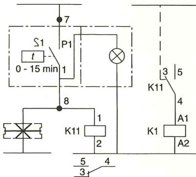
Valojen/hälytyksen ja kontaktorin vaihto-ohjaus kylmähuoneessa.
