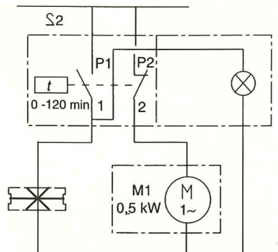
Valojen/hälytyksen ja puhaltimien suora vaihto-ohjaus.
