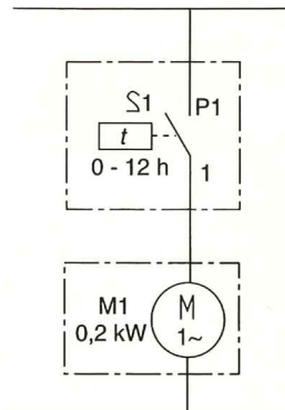
Lämpöpuhaltimen tai vastaavan ohjaus aikakytkimellä.
