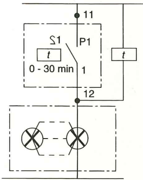
Siivouskytkimenä porraskäyttö-automatin ohituksessa.
