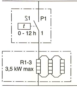
Säteilylämmittimen ohjaus
