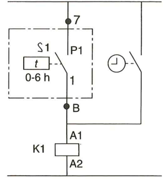
Ilmastoinnin kello-ohjaus, jossa aikakytkinohitus.
