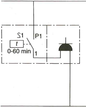
Keittiön pistorasian ohjaus vanhustentalossa.
