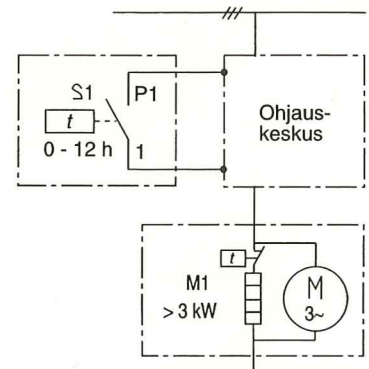
Ovipuhaltimen paikallisohjaus.
